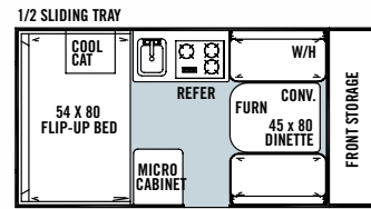
1/2 SLIDING TRAY RVQUE GAS GRILL
